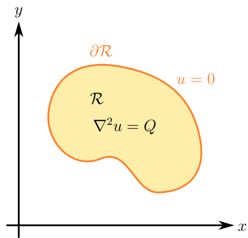
Slika 1: Poissonova enačba s homogenimi robnimi pogoji.
